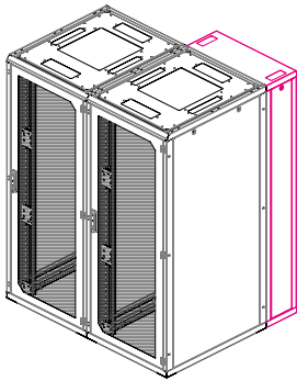
Section avant/arrière
