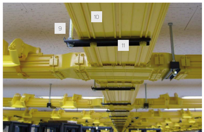
2. Installation d'OptiWay au plafond
