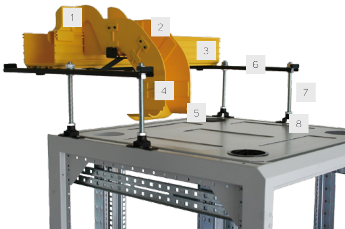
1. Installation d'OptiWay en haut de la baie
